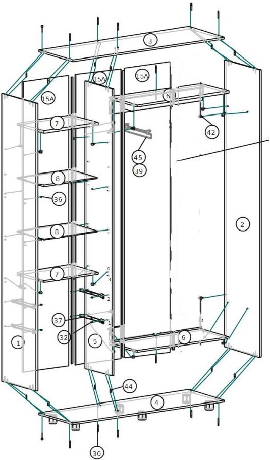
Рис.5 Сборка корпуса
