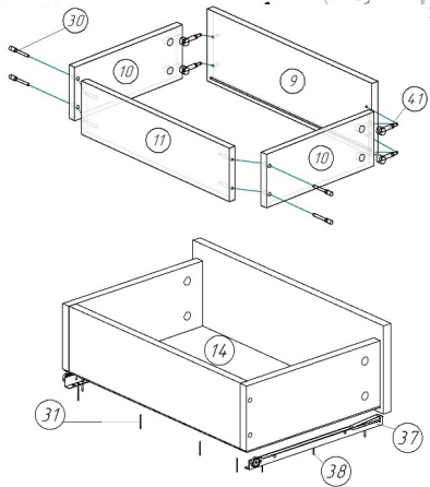
Рис.3 Схема сборки на эксцентриковую усиленную стяжку (42)
